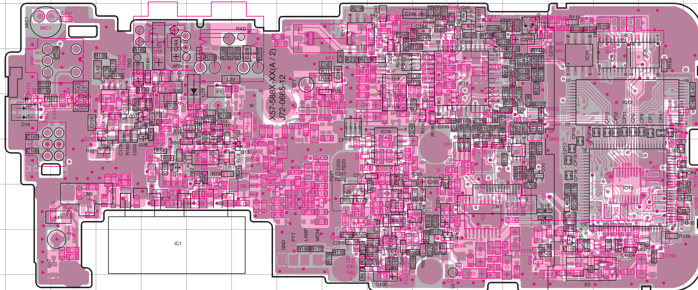
Ref. NO. Address Ref. NO. Address IC1 8E Q21 8N IC2 7H Q22 3J IC3 6F Q23 3L IC4 4J Q24 5C IC5 4O Q25 5B IC6 4P Q26 8K IC7 8P Q27 8O IC8 5P Q28 8O IC9 6D Q30 4E IC10 4N Q31 8N IC11 5D Q32 5D IC12 5O Q33 5D IC13 7O Q34 5E IC14 4L Q35 3L IC15 6M Q36 6M IC16 7K Q301 5N IC17 3I D1 7K IC18 6J D2 7J IC19 8J D3 7D Q1 8K D4 7J Q2 7I D5 6H Q3 7I D6 6J Q4 7H D7 6J Q5 7H D8 7E Q6 7H D9 8J Q7 6I D10 6H Q8 6J D11 8K Q9 6F D12 6J Q10 8J D13 4K Q11 6J D14 4I Q12 5K D15 5F Q13 6G D17 7M Q14 5K D18 5B Q15 6E D19 7M Q16 8M D21 7P Q17 5K D22 4F Q18 8N D23 3M Q19 5H D302 6G Q20 8N D305 5E D306 5E D307 5O
