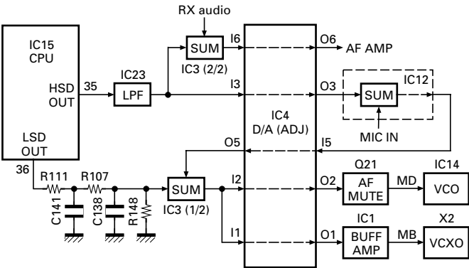
Fig. 12 Encode
