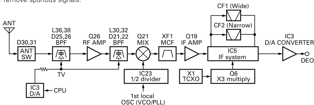
Fig. 2 Receiver system / 图2 接收部系统
