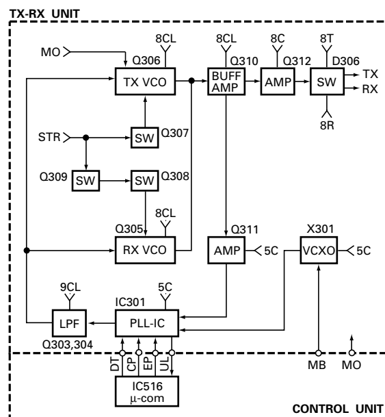
Fig. 9 VCO/PLL circuit
