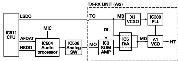
Fig. 13 Encode
