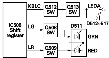
Fig. 11 Display circuit
