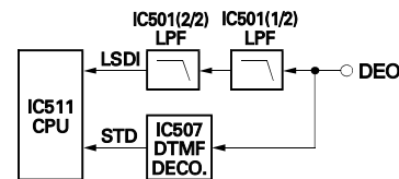
Fig. 14 Decode
