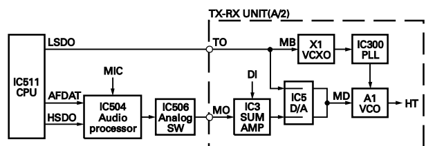
Fig. 12 Encode
