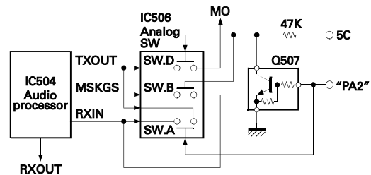
Fig. 15 PA switch
