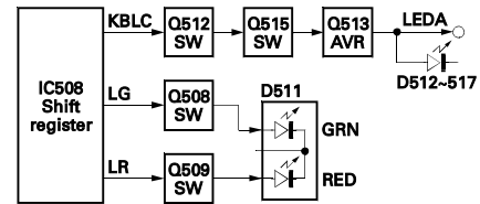
Fig. 10 Display circuit
