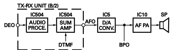
Fig. 3 AF signal system
