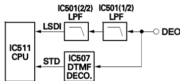
Fig. 13 Decode
