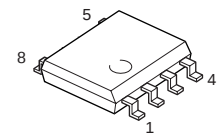
NJM4558E
