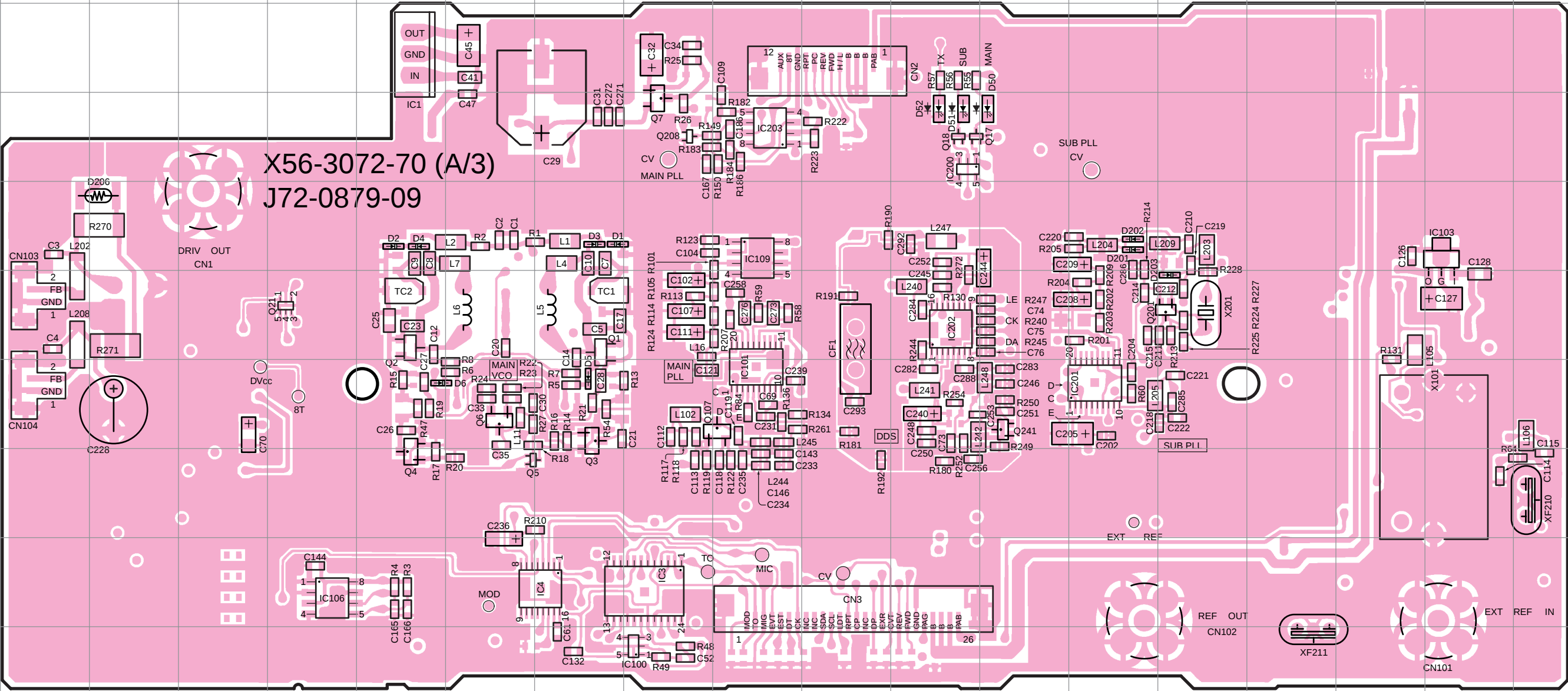
TX UNIT (X56-3072-70) (A/3) Component Side View (J72-0879-09)
