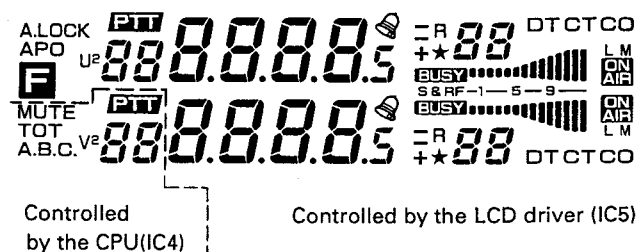
Fig. 16 Display LCD
