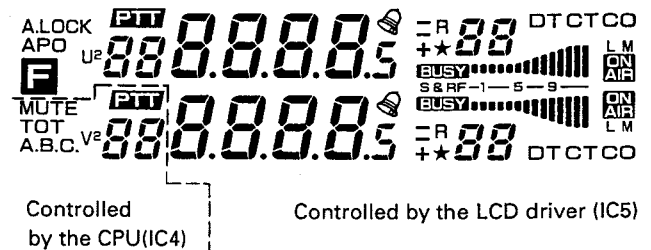
Fig. 16 Display LCD
