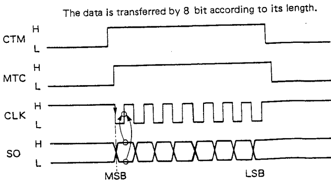
Fig. 12 Timming chart
