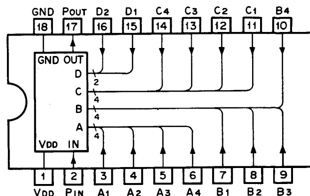
Fig. 5 TC9122P (PLL Unit : Q18)
