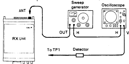
Fig. 20 RX 2. Helical
