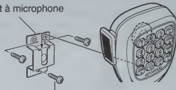
Vis pour crochet à microphone (3 mm x 10 mm)
