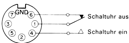
REMOTE-Buchse (von der Rückwand aus gesehen)
