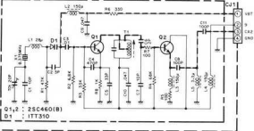
CAR-2 UNIT (X50-1460-00)
