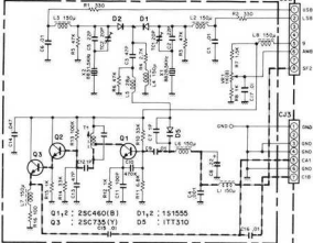
CAR-2 UNIT (X50-1460-00)
