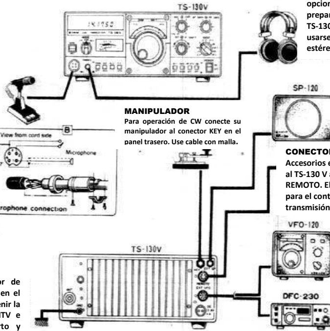
Fig. 2-2 [A] TS-130V Interconexión
