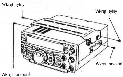
Wkręt przedni
