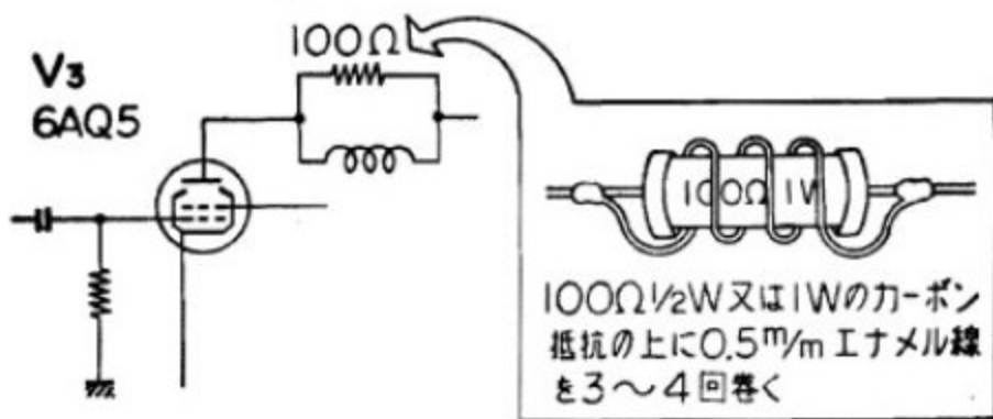
〔第3図〕 パラドメの作り方
