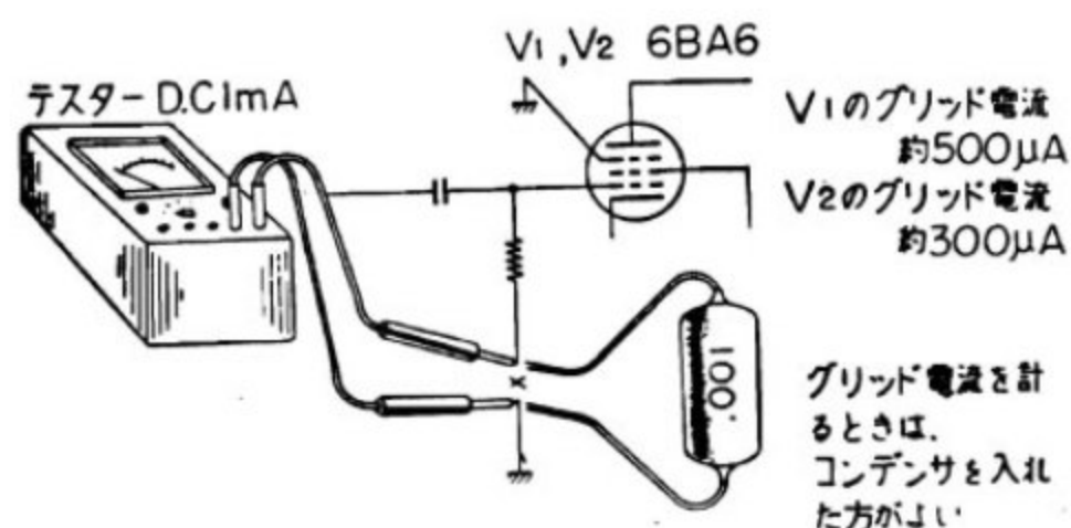
〔第2図〕グリッド電流の計り方(発振の確認)
