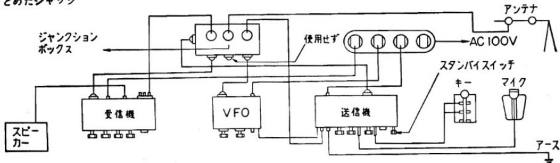
〔第6図〕 ジャンクション・ボックスを使ったシヤック
