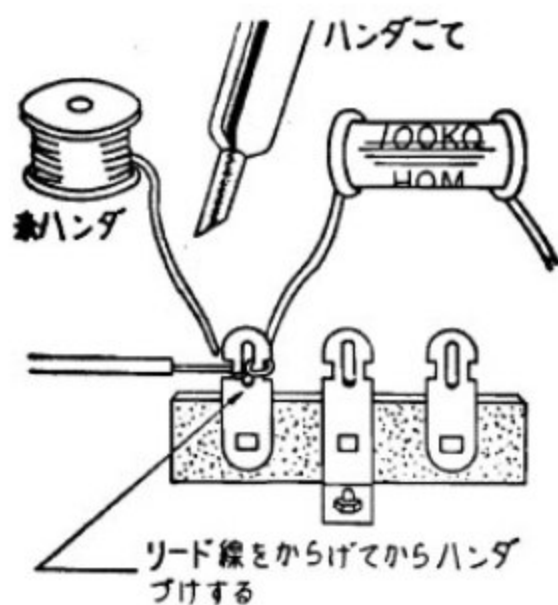
〔第2図〕ハンダづけのし方
