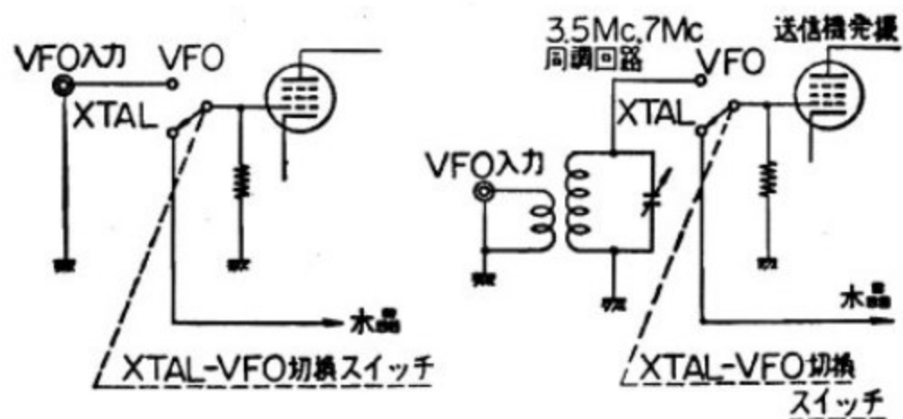
〔第4図〕 送信機へのつなぎ方 〔第5図〕
