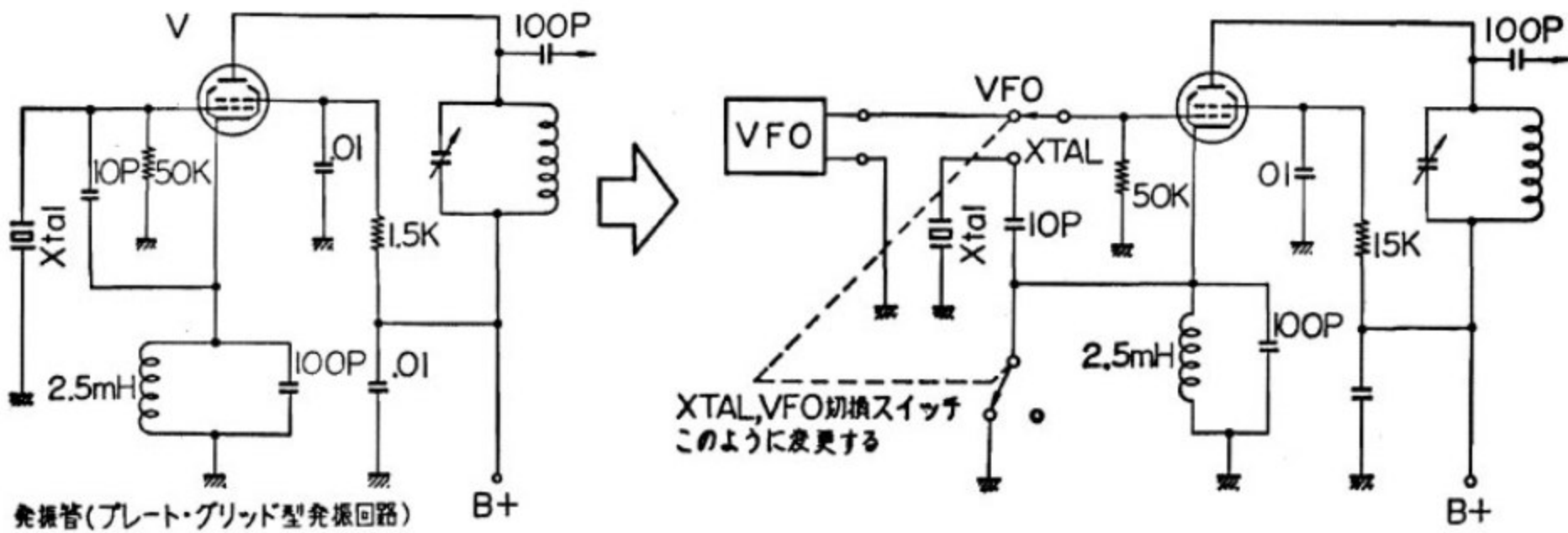
〔第4図〕 VFO のつなぎ方
