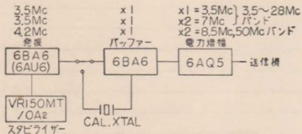
〔第1図〕VFO-1のブロックダイヤグラム
