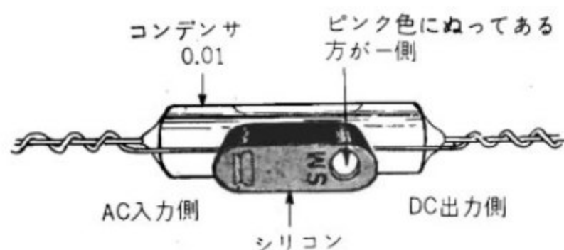
〔第1図〕シリコン整流器の極性
