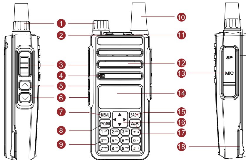
Bild 2.1. Radioddity GA-510, übersicht
