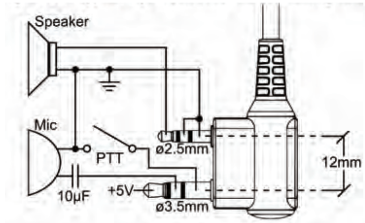
Bild 2.3. Typische 2-pin Kenwood Headset Konfiguration.
