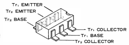
IMB6 (B6) (Q2014)
