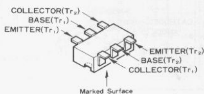
IMD2(D2) (Q1006, 1012)
