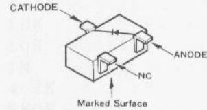
1SS153(A9) (D304)
