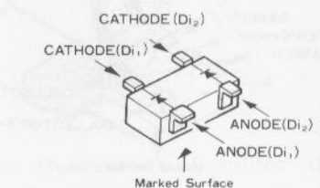
1SS319(A4) (D1006)
