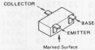
2SC3356(R24) (Q301)
