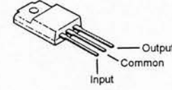
KIA7805PI (Q6001)
