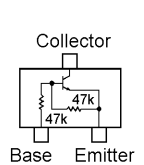
RT1N441U (N3) (Q1042, 1053)
