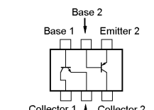
IMZ2 (Z2) (Q1057)
