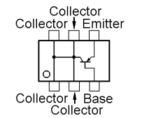
CPH6102 (AB) (Q1051)
