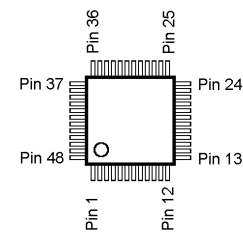
LC75834W (Q1054)
