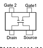
SGM2016AM (MA) (Q1026)
