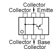
CPH6102 (AB) (Q1029, 1031)
