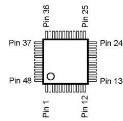
M37516E6HP (Q1014)
