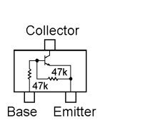
RT1N441U (N3) (Q1042, 1053)
