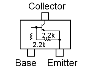
DTB123EK (F12) (Q1036)
