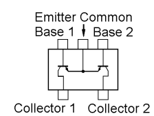
FMW1 (W1) (Q1032)
