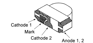
12-22SURSYGC/S530-A2/TR8 (D1026)
