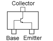
2SC4154E (LE) (Q1008, 1055) 2SC5005 (73) (Q1007) 2SC5006 (24) (Q1012) 2SC4215Y (QY) (Q1033) 2SC5227 (LN) (Q1015)
