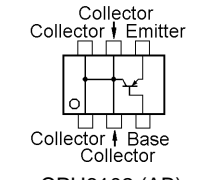
CPH6102 (AB) (Q1029, 1031)
