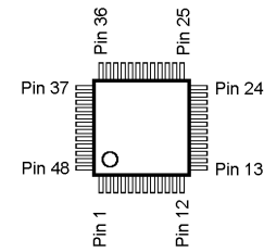
LC75834W (Q1054)
