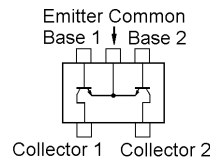
FMW1 (W1) (Q1027, 1028)
