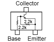
DTB123EK (F12) (Q1036)
