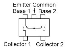
FMW1 (W1) (Q1027, 1028)
