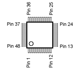
M37516E6HP (Q1014)
