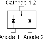
DAN235E (M) (D1014)
