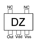
S-80735SN (DZ) (Q1041)
