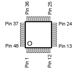
M37516E6HP (Q1014)
