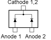
DAN235E (M) (D1014)
