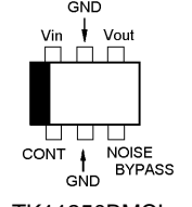
TK11250BMCL (Q1040)
