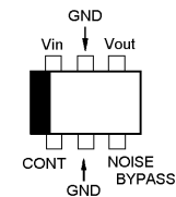
TK11250BMCL (Q1040)
