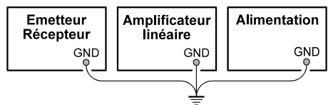
Branchement de mise à la terre correcte
